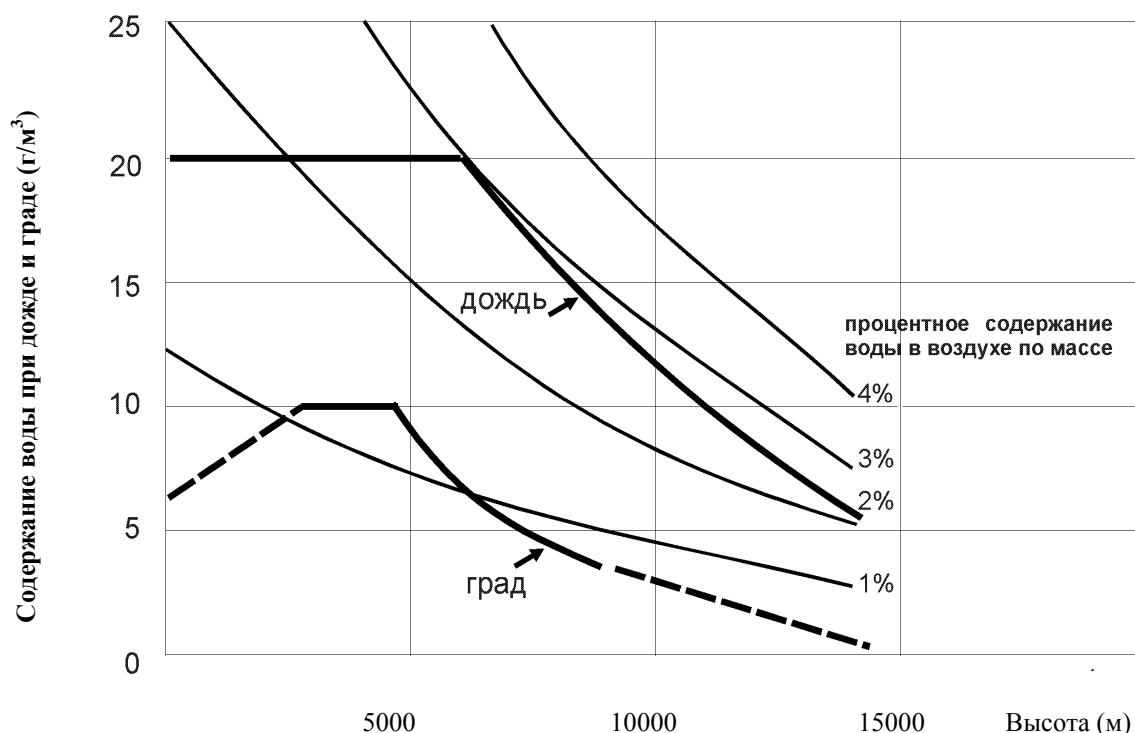
Рис.В1. Содержание воды при дожде или граде (г/м³)
